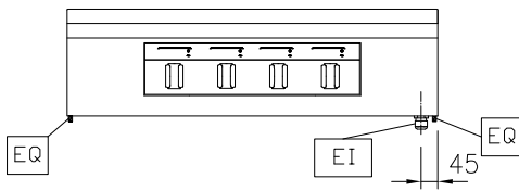
Front aanzicht
