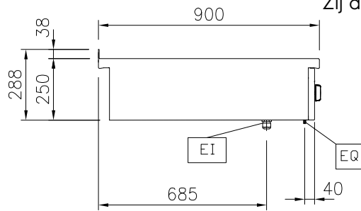
Zij aanzicht
